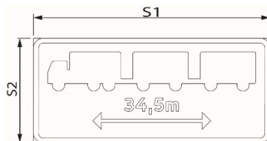
Storlek och mått i meter för märke F31a
