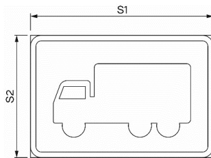
Storlek och mått i meter för märke F31
